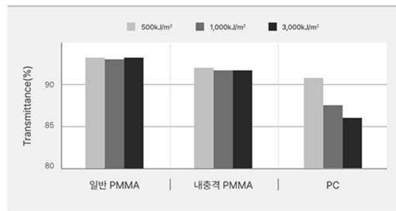
UV 노출에 따른 투과율 변화
