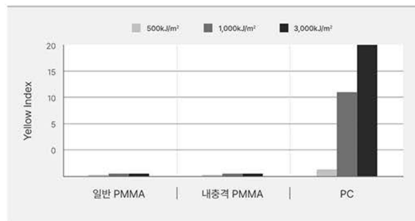
UV 노출에 따른 YI 변화
