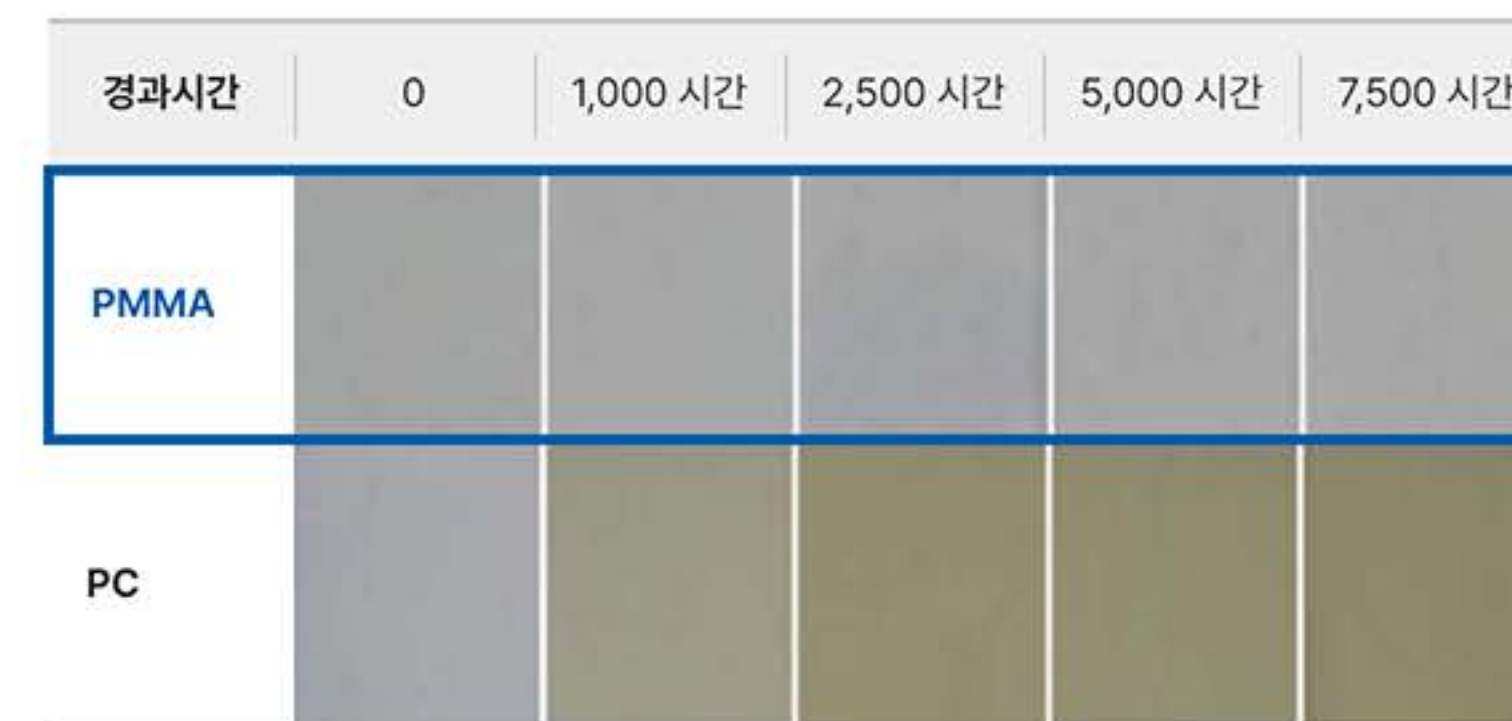
촉진 내후성 테스트 후 시편 변화
